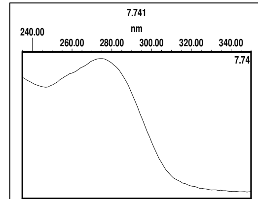
Isoadhumulone
